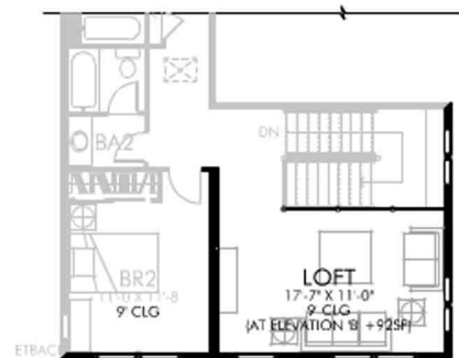
UPPER LEVEL OPTIONAL 'B' ELEVATION
